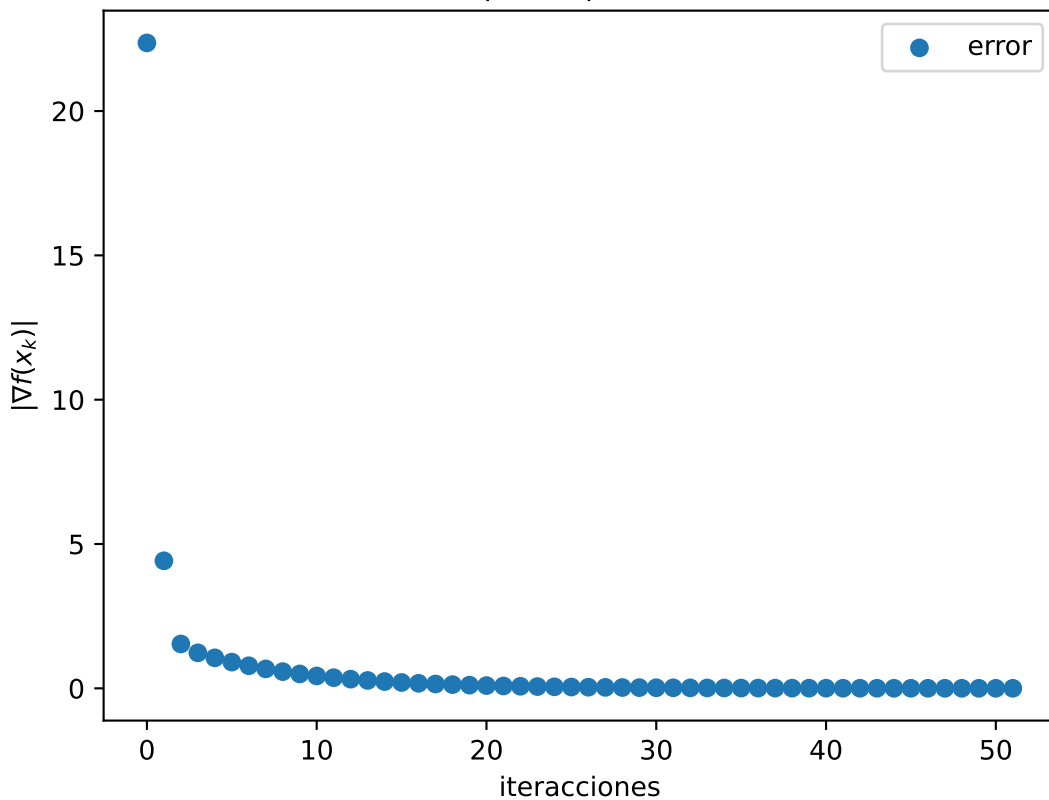
Gráfica |\nabla f(x_k)| de funcion ii
